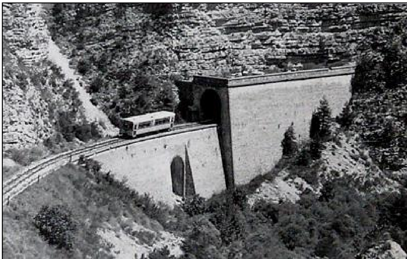
Vue de l'entrée du tunnel de Méailles protégée par une galerie artificielle
