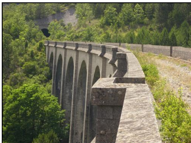
La sortie du tunnel suivie du viaduc de Caylaret
