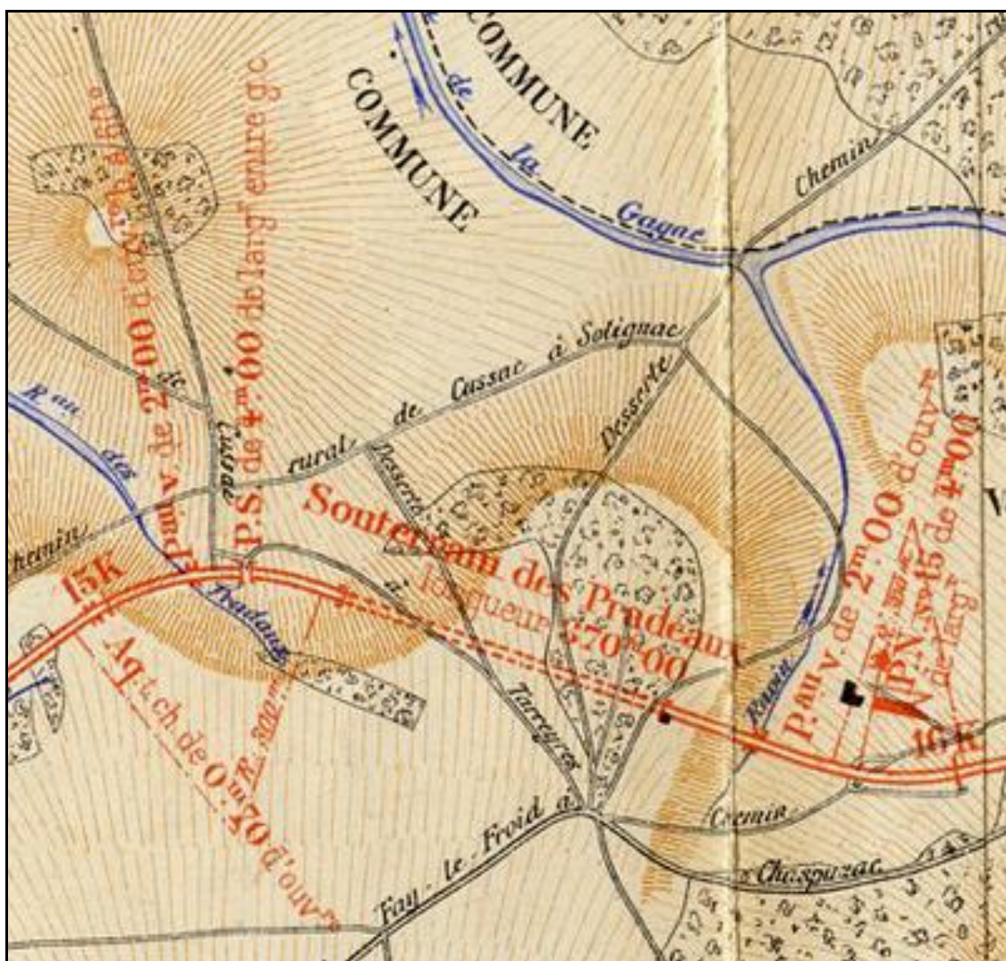
Plan d'époque du tunnel des Pradeaux
