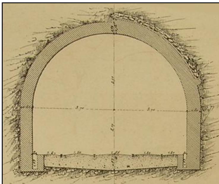
Ci-dessus et ci-dessous, coupe et divers aspects de la galerie du tunnel de Rilly
