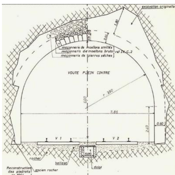
Deux coupes de la galerie du tunnel de Nouaillas 2
