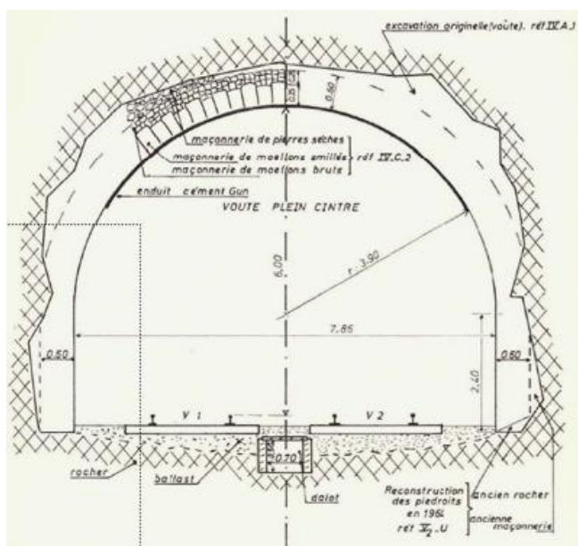
Deux coupes de la galerie du tunnel de Nouaillas 2
