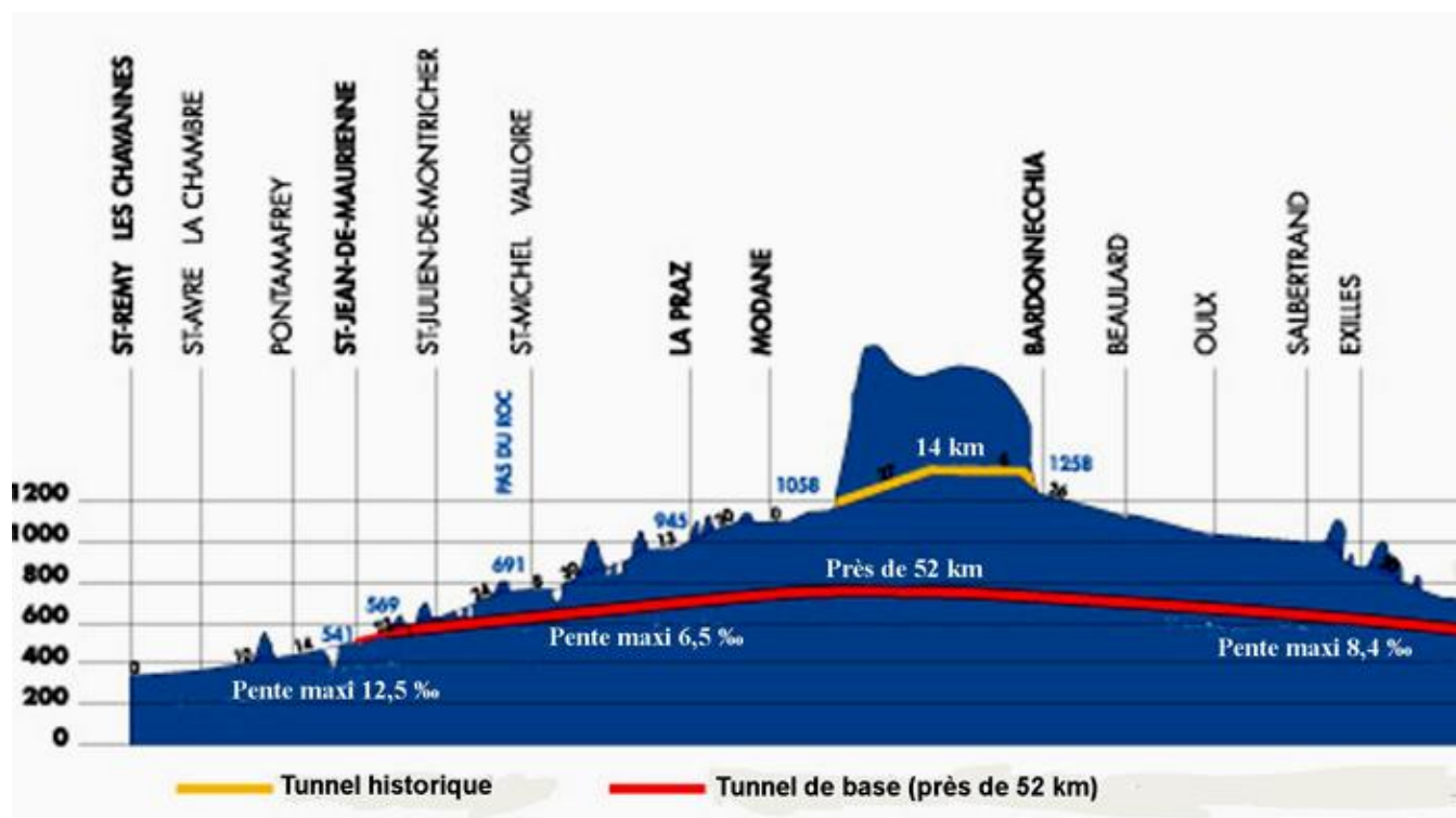
Ci-dessus et ci-dessous, coupes du massif alpin et du tunnel
