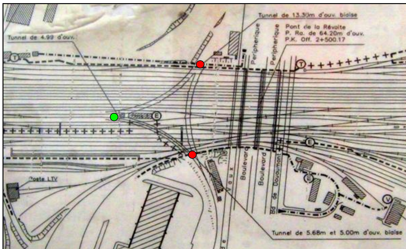
Plan de l'ouvrage sous les voies principales de la gare Saint Lazare Batignolles Attention, sur ce croquis, le nord est en bas du dessin
